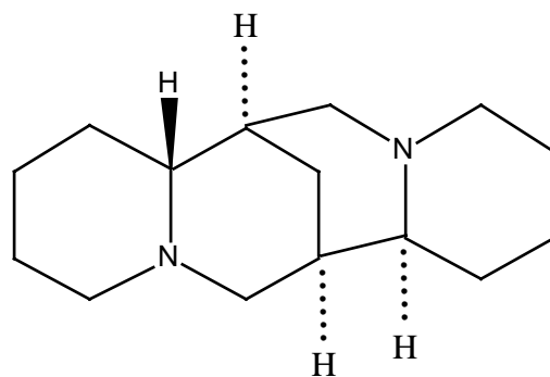
(-) Sparteine
