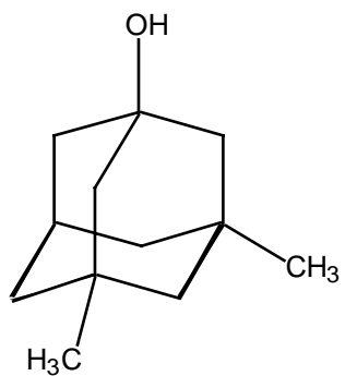
3,5-Dimethyl-1-adamantanol
