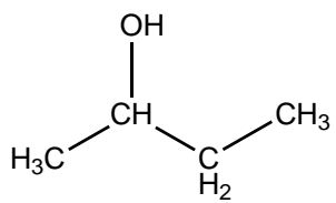
2-Butanol
