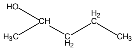
2-Pentanol
