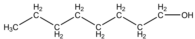
1-Octanol
