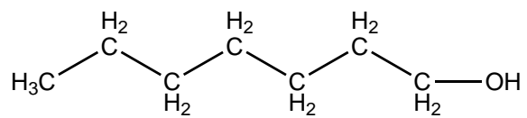
1-Heptanol
