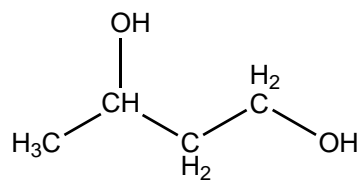
1,3-Butanediol
