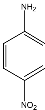
4-Nitroaniline
